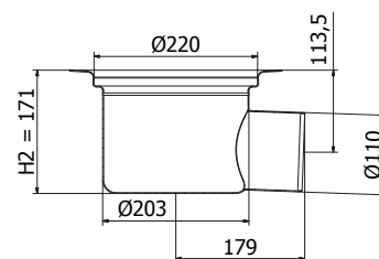
Sida Ø110 mm (Syrafast rostfritt stål)
